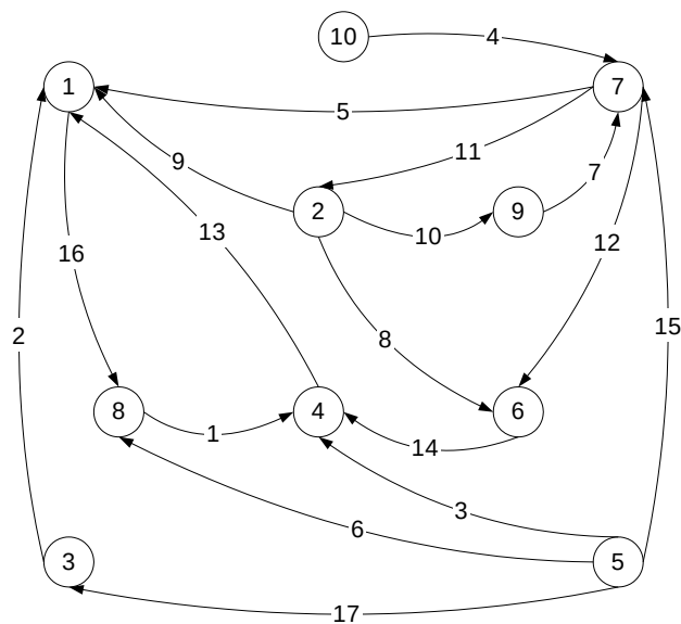
Рис. 1.5. Диаграмма орграфа
