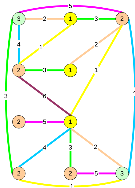
Рис. 1.4 Раскраска графа
